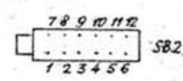
Схема нумерации выводов переключателей (вид со стороны печатного монтажа)
