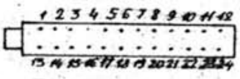
Схема нумерации выводов переключателей (вид со стороны печатного монтажа)
