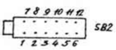
Схема нумерации выводов переключателей (вид со стороны печатного монтажа)
