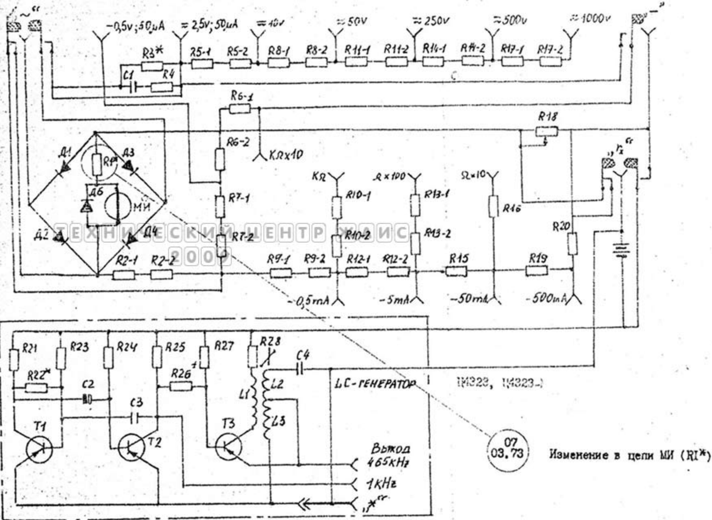
Схема электрическая принципиальная с 07.1972 г.
