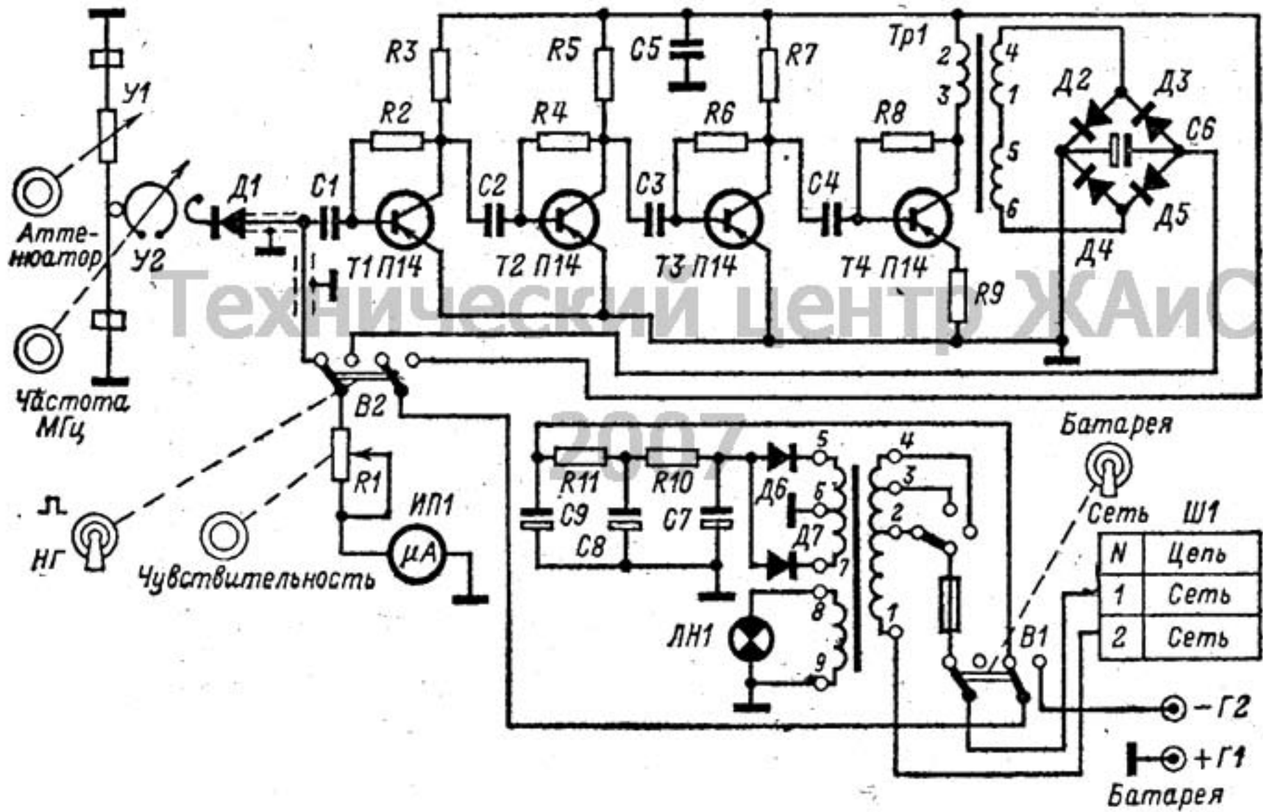
Электрическая принципиальная схема резонансного частотомера Ч2-32.
