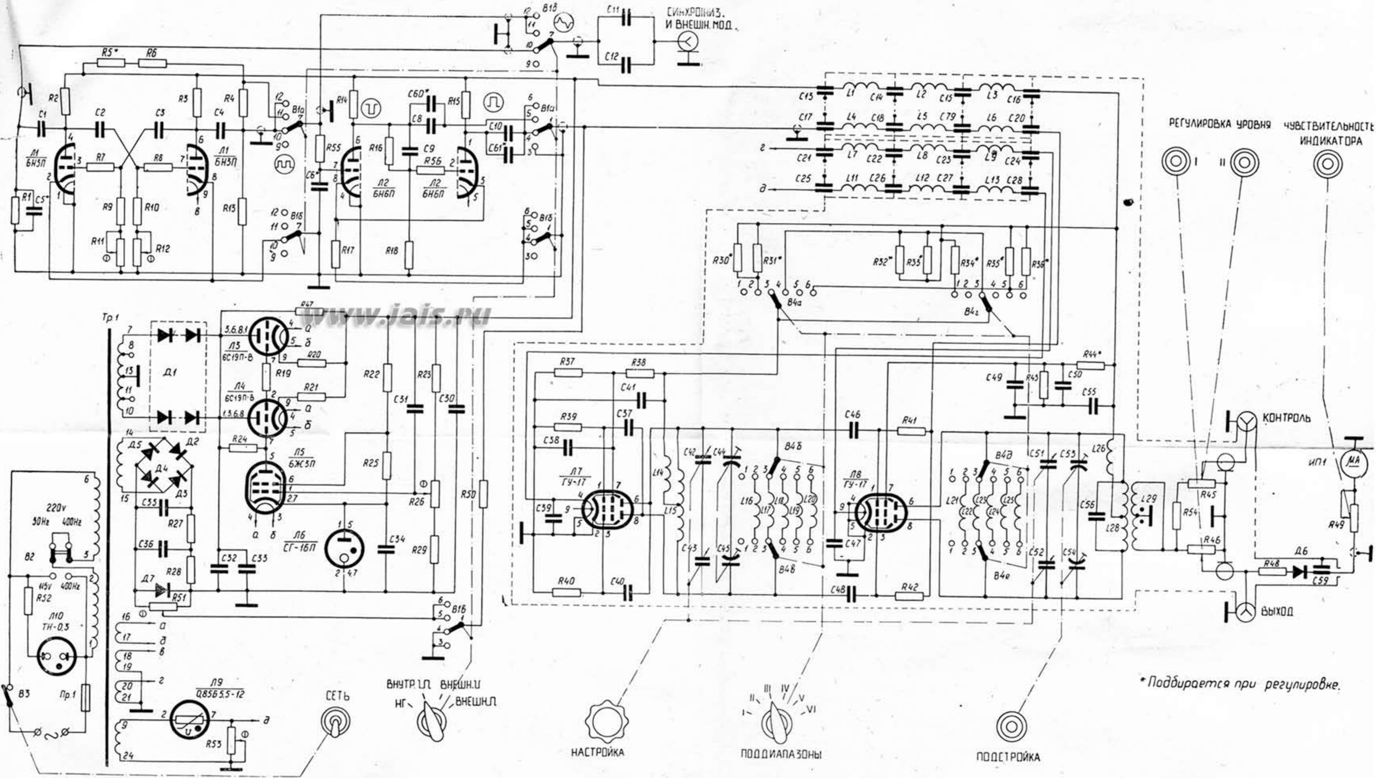
Принципиальная схема ГЗ-19А.
