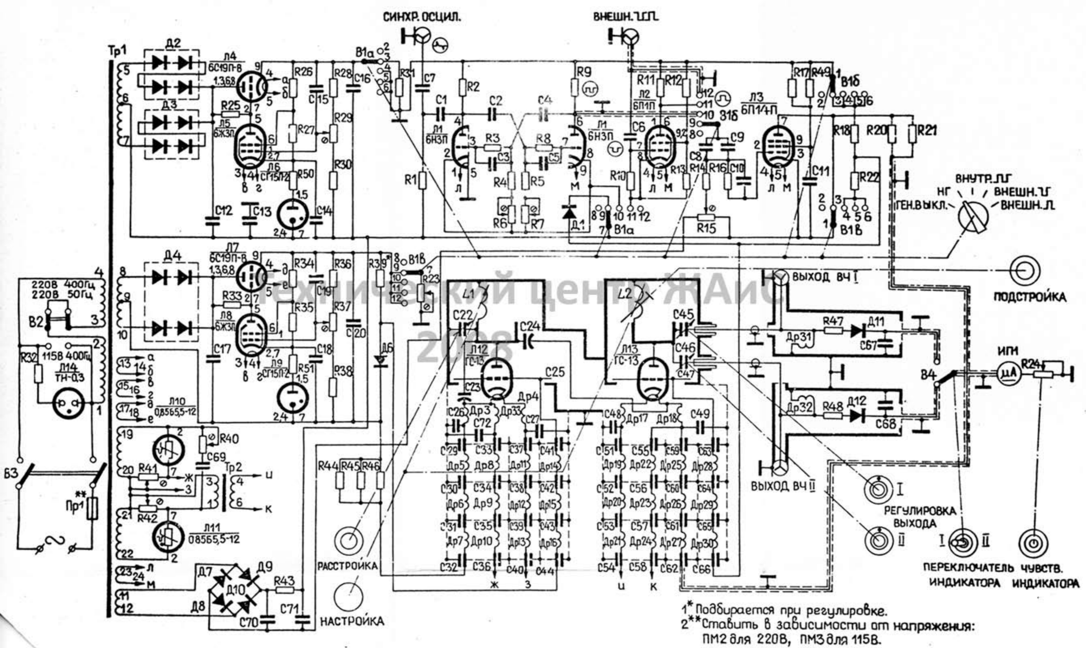
Рис.1. Генератор сигналов Г4-120. Схема электрическая принципиальная.
