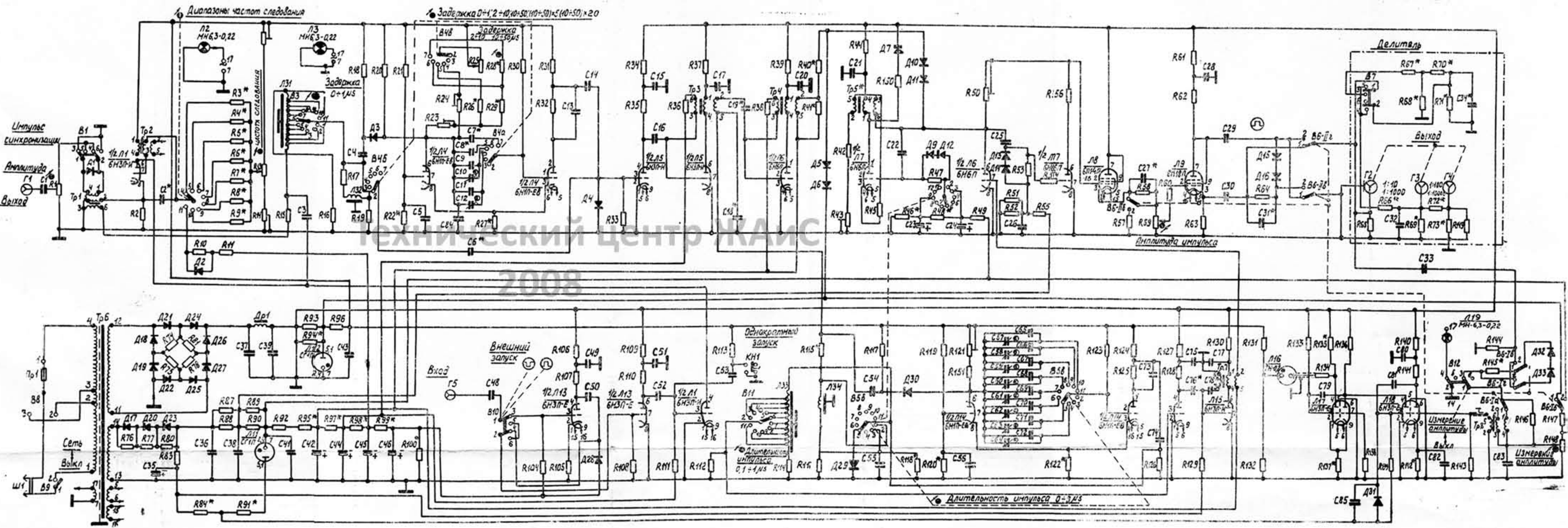
Принципиальная электрическая схема.
