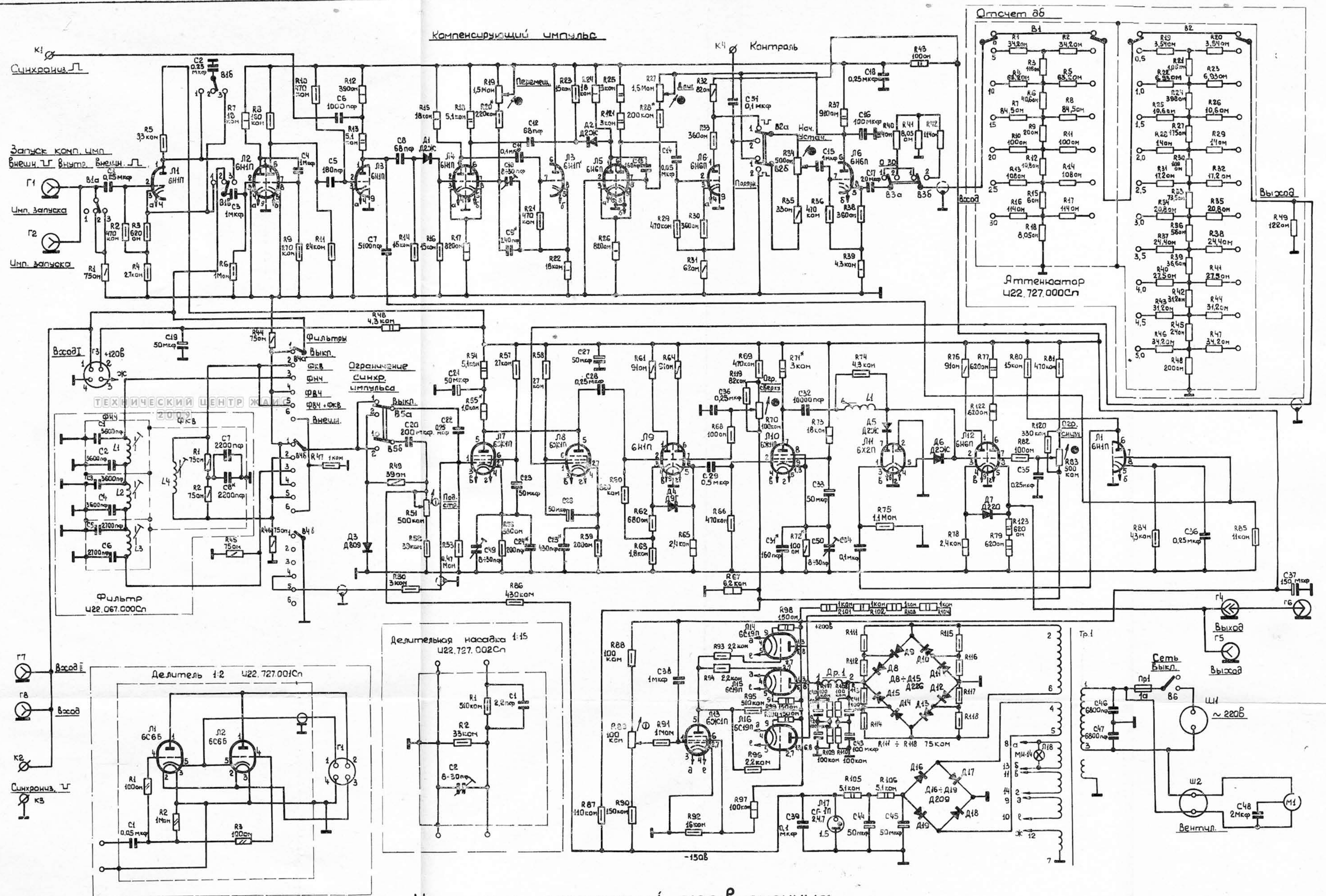
Измеритель искажений телевизионных испытательных сигналов.
