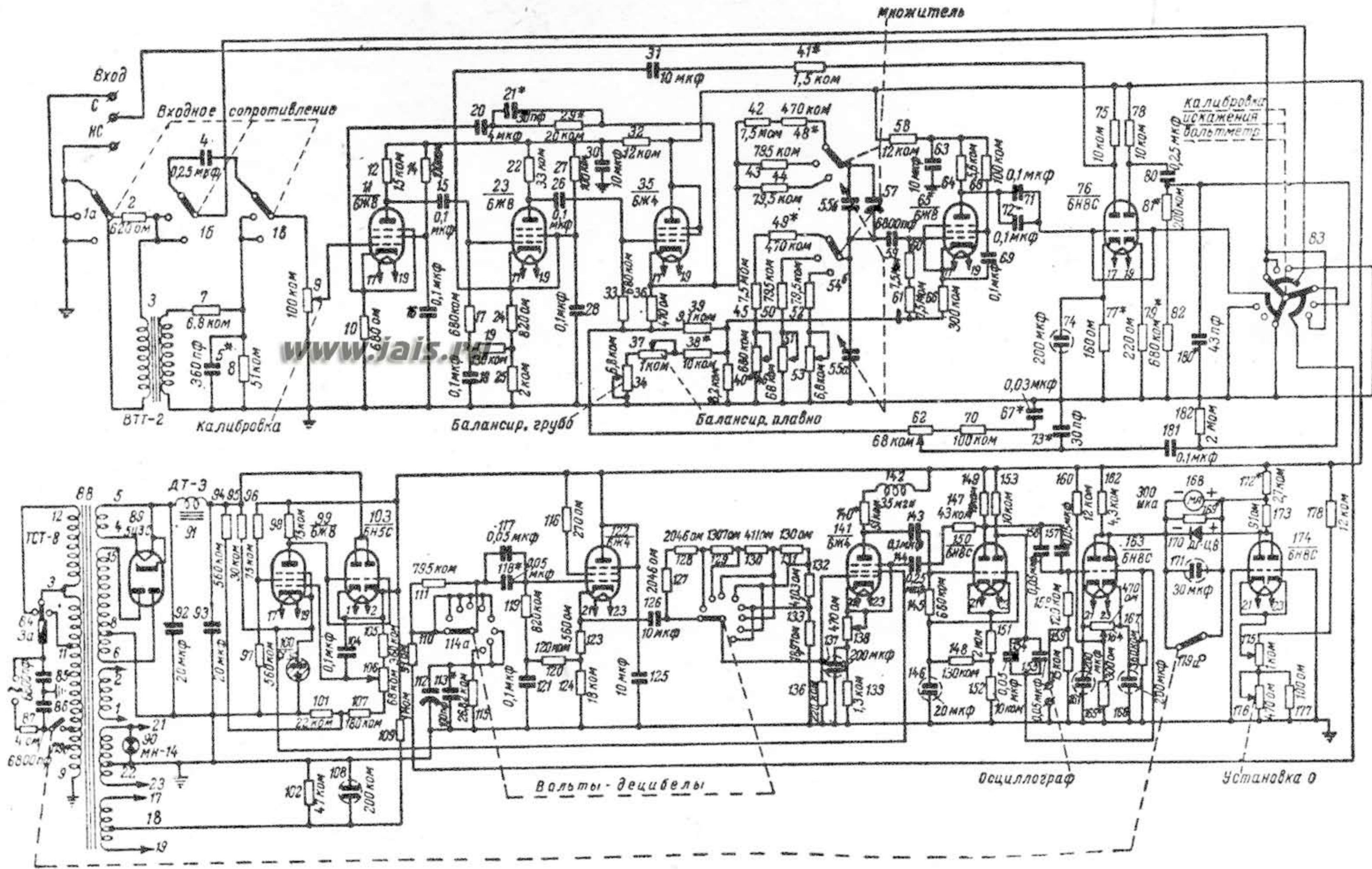
Рис. IV. Принципиальная схема измерителя нелинейных искажений ИНИ-11.
