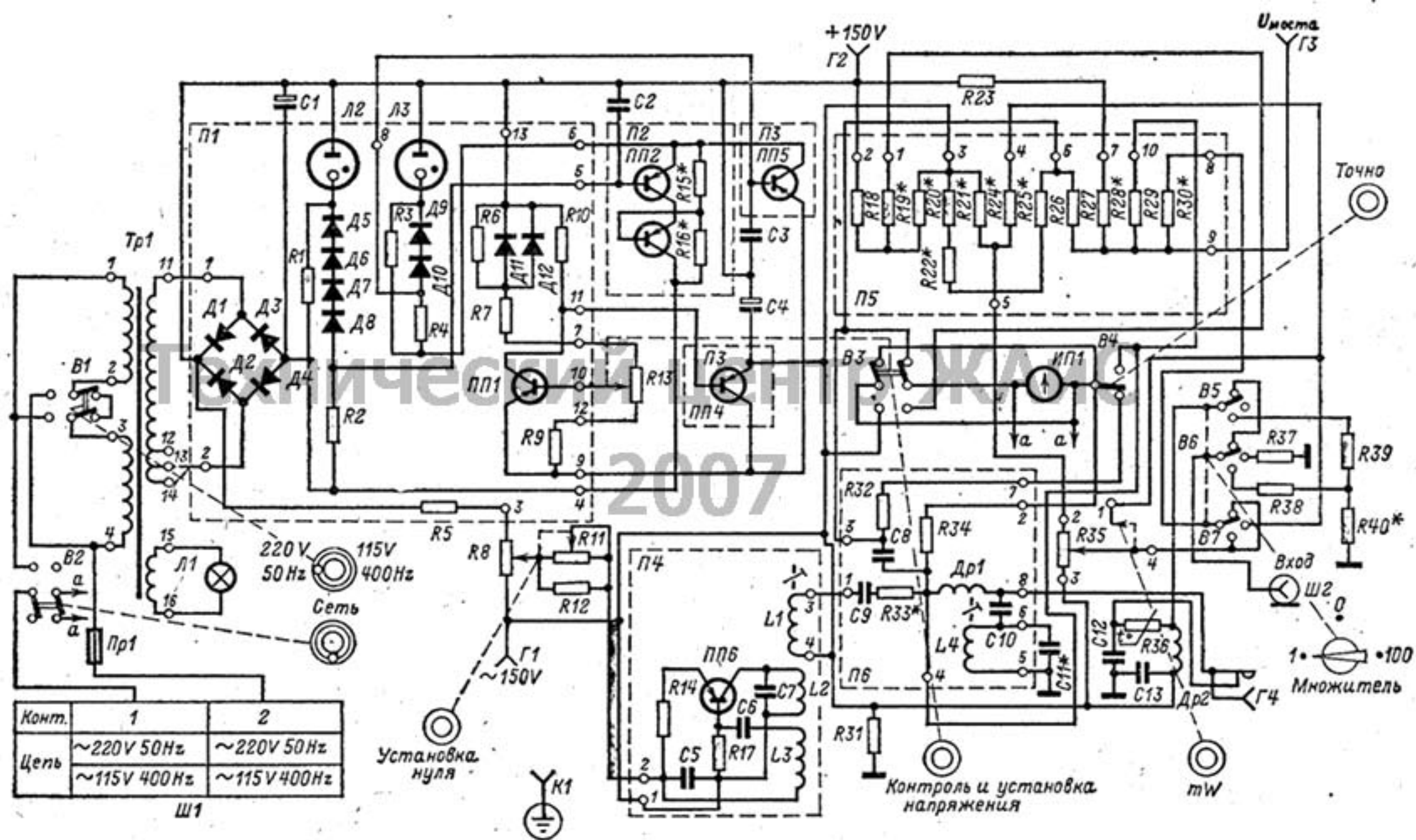
Электрическая принципиальная схема измерителя малых мощностей МЗ-1А.
