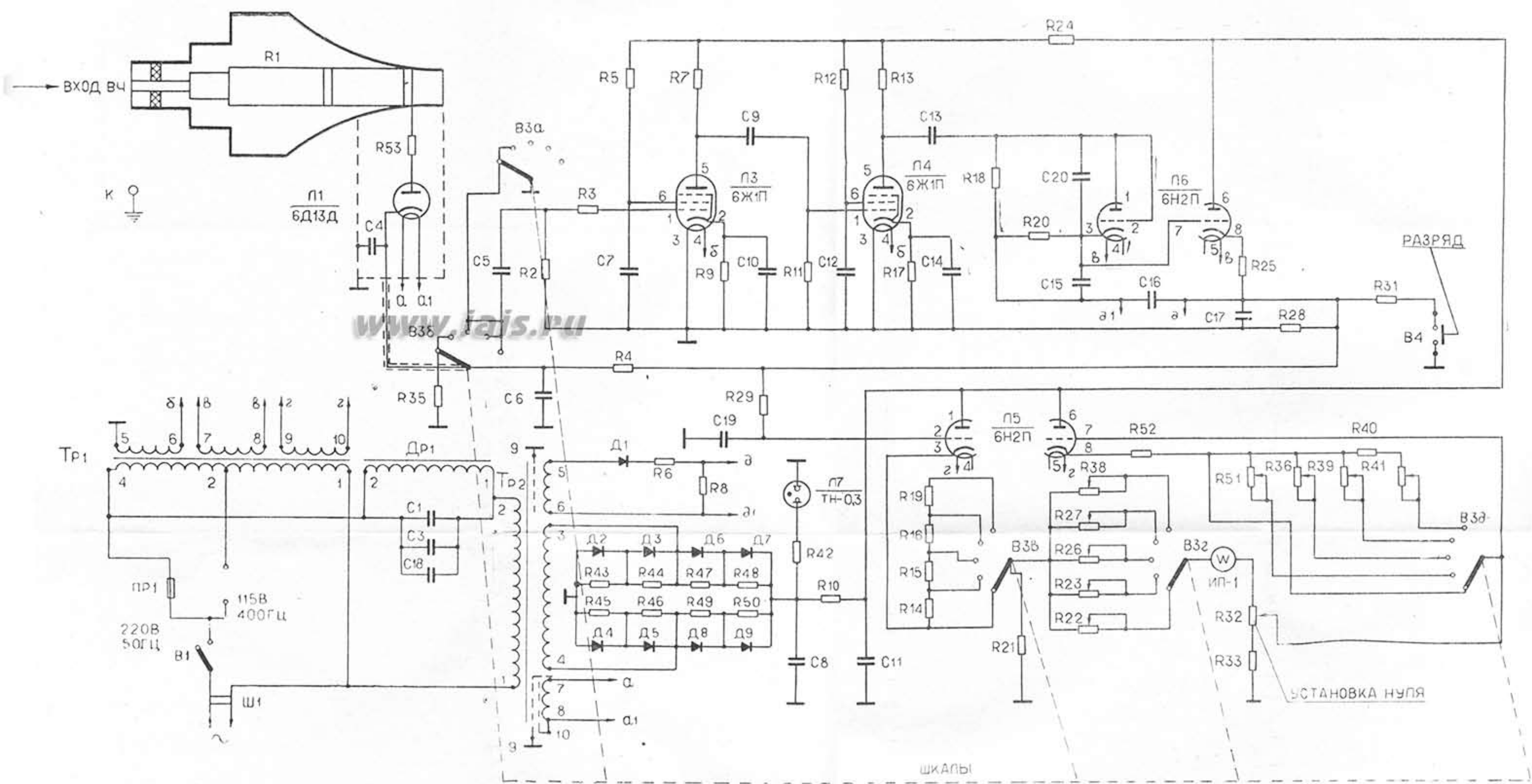
ЧЕРТ 2 ПРИНЦИПАЛЬНАЯ СХЕМА ПРИБОРА ТИПА М3-3А
