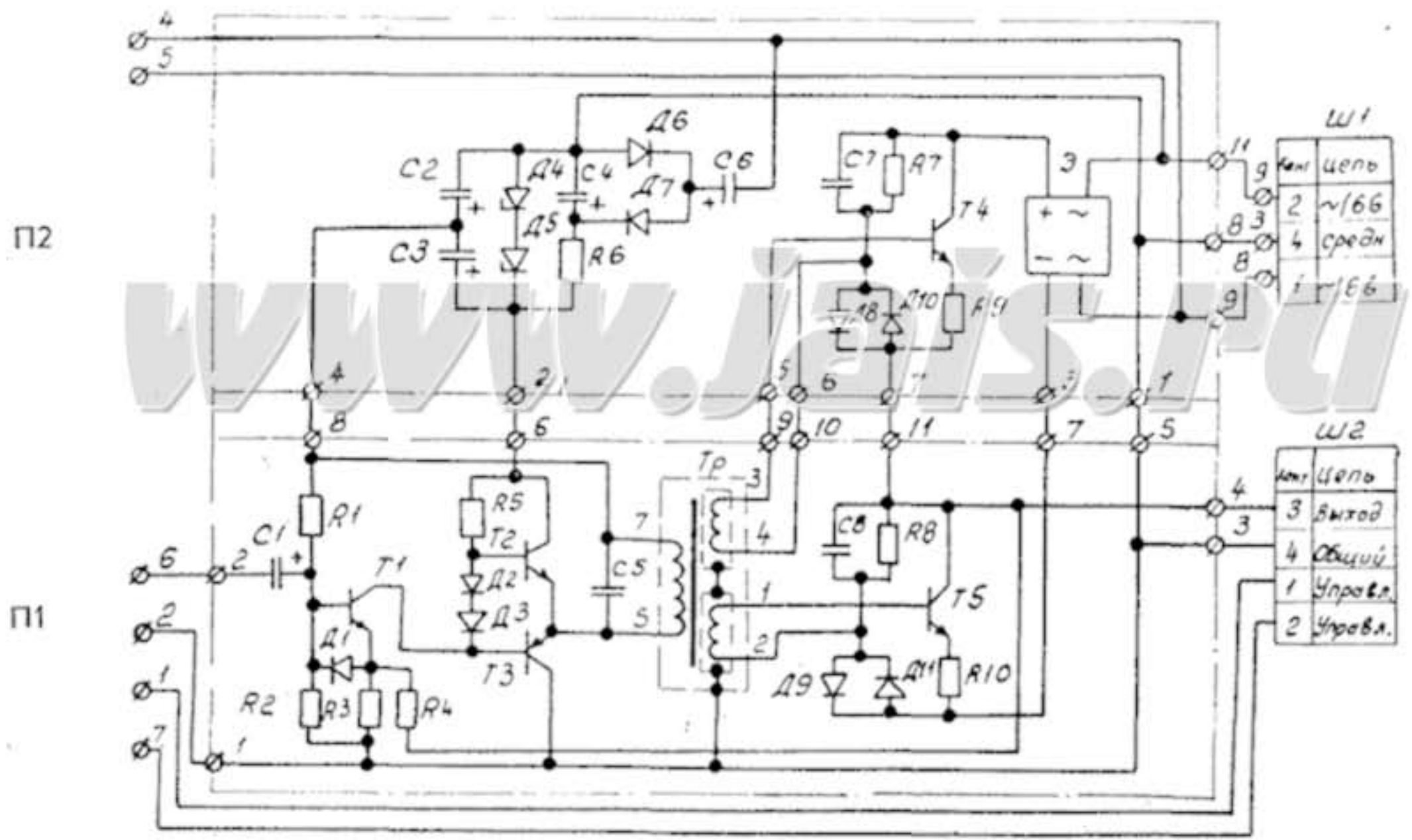
Усилитель окончательный
