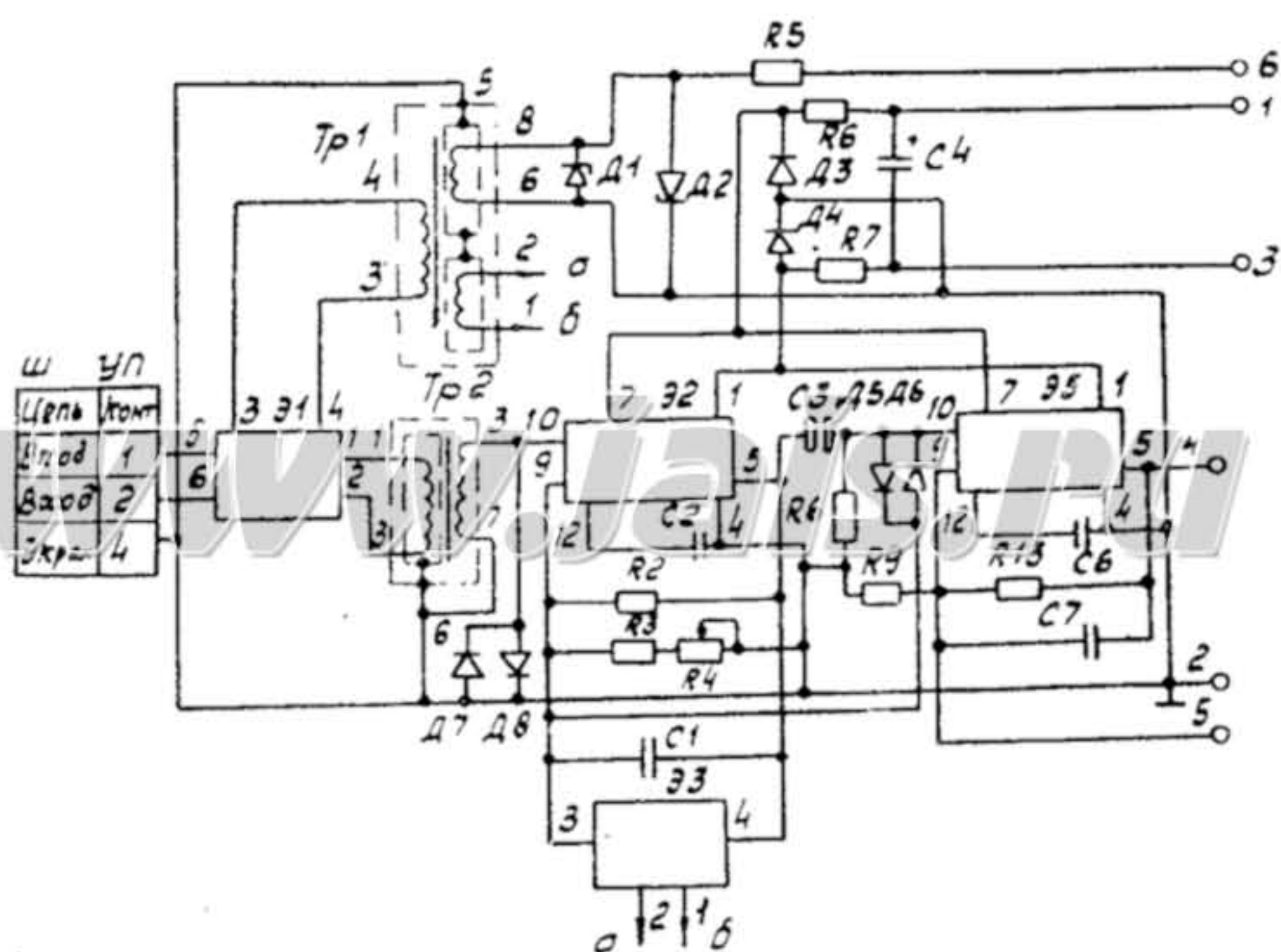
Усилитель предварительный
