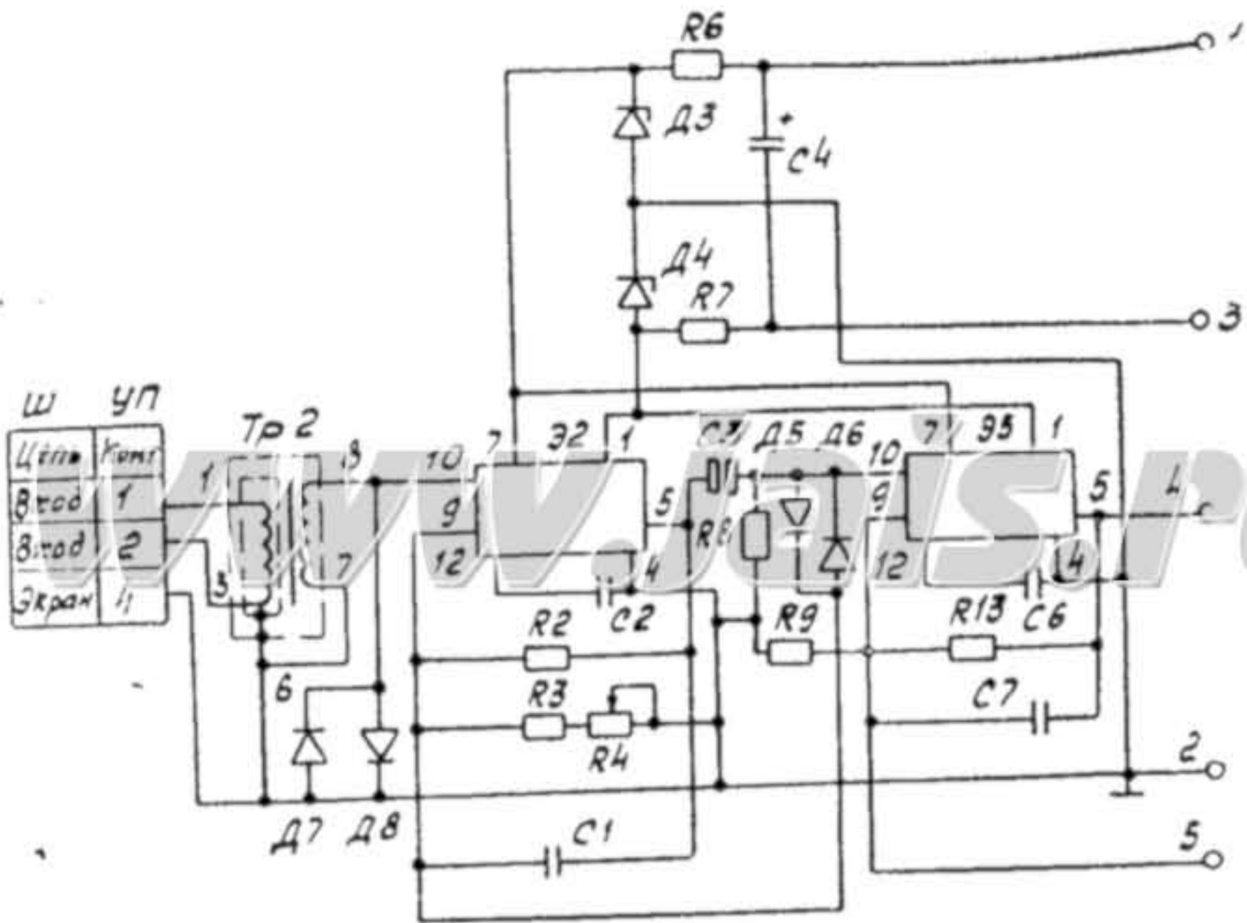
Усилитель предварительный
