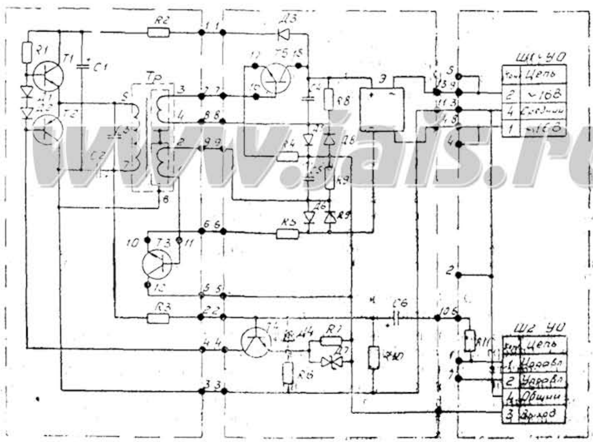
Усилитель оконечный
