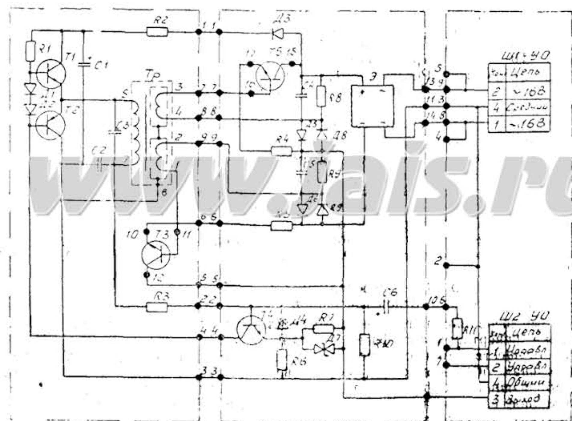
Усилитель оконечный
