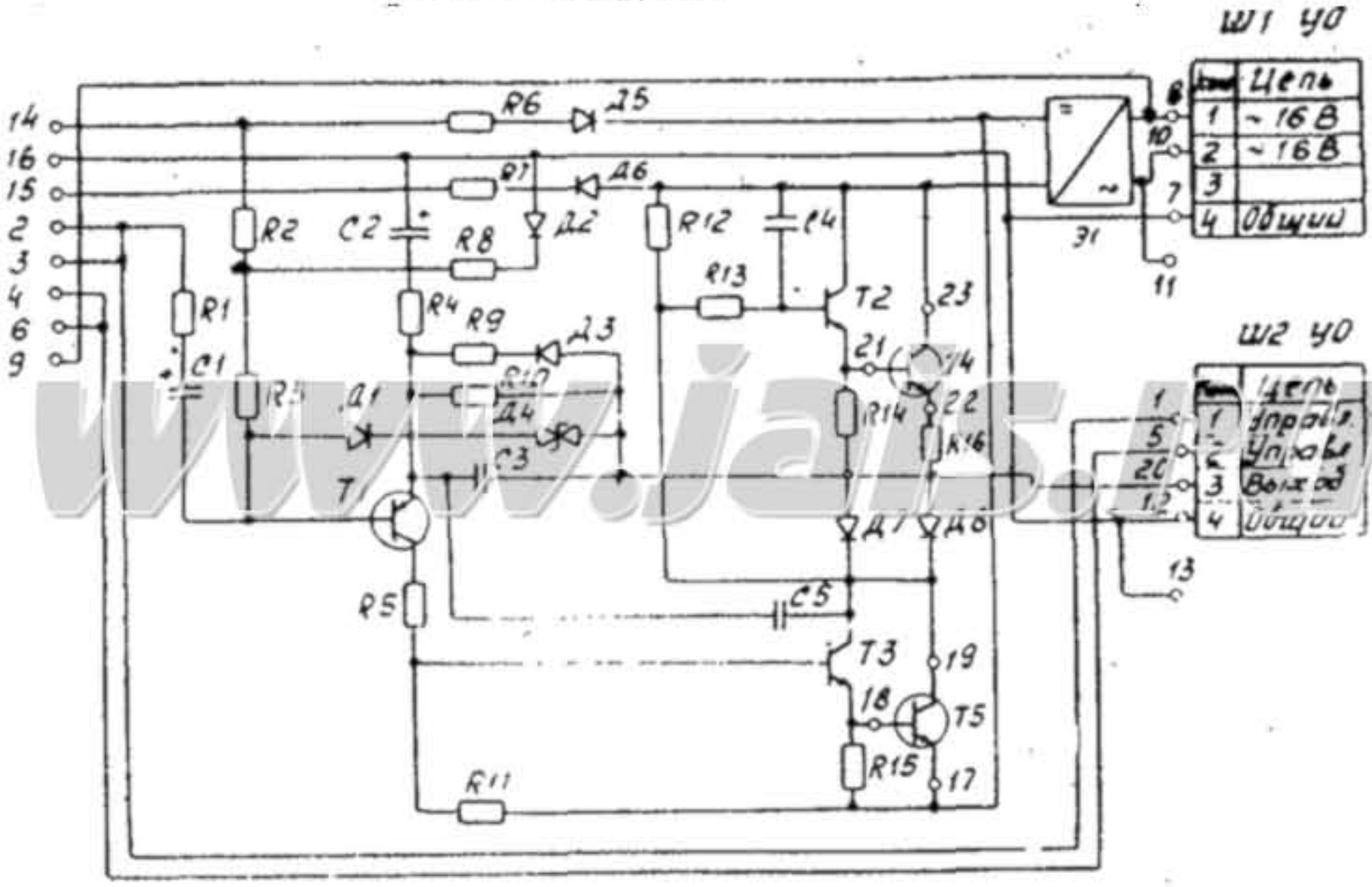
Усилитель оконечный
