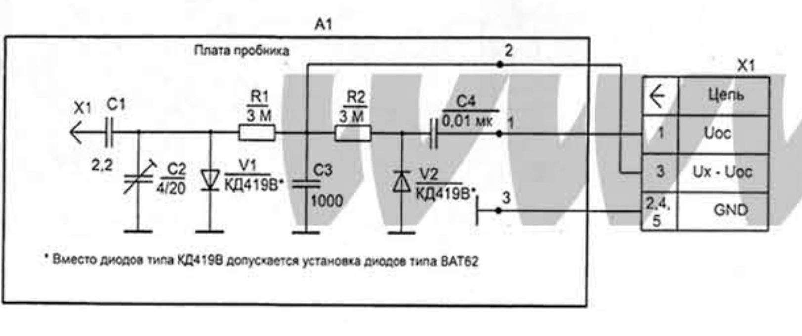
ПРОБНИК 1:10. Схема электрическая принципиальная
