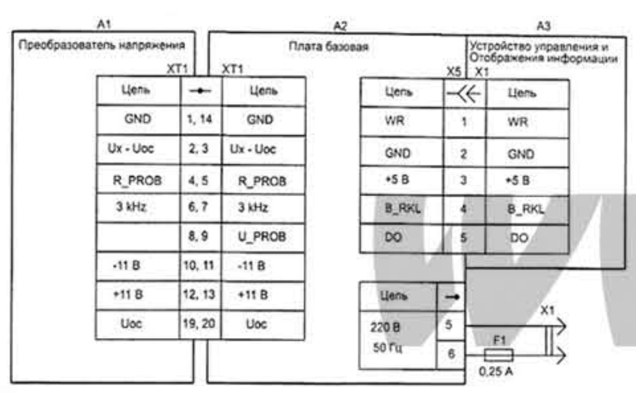
ПРОБНИК 1:1. Схема электрическая принципиальная
