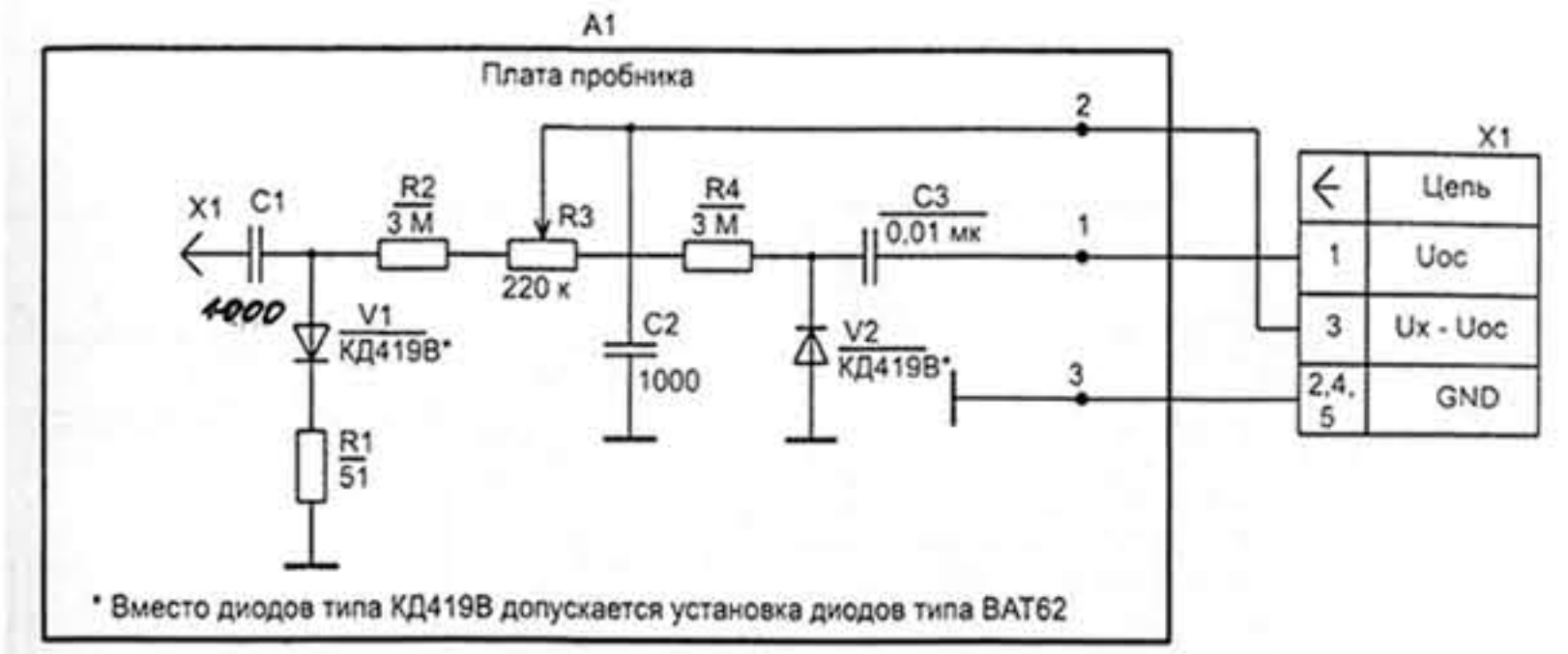
ПРОБНИК 1:1. Схема электрическая принципиальная
