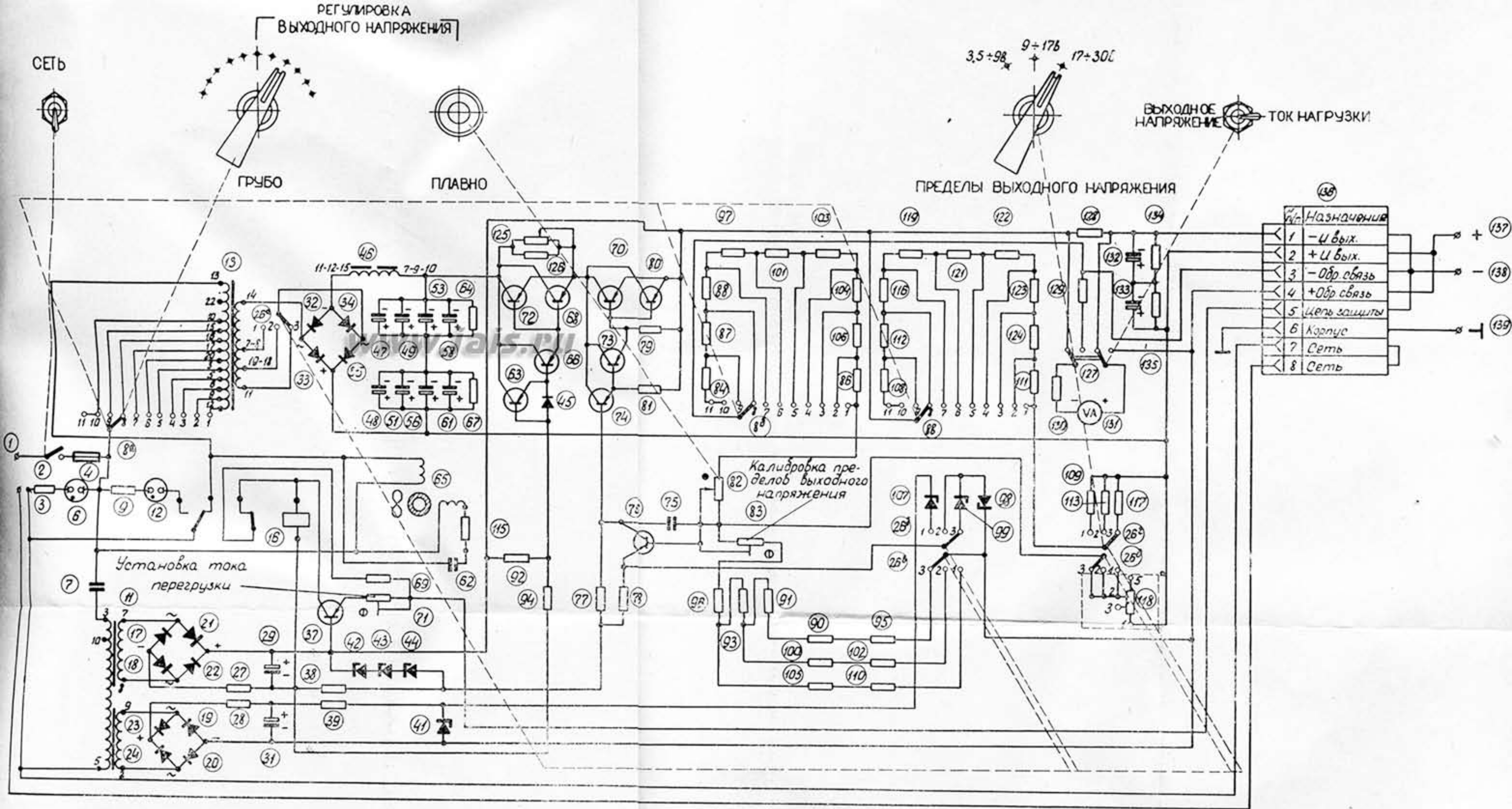
И.5. Схема принципиальная электрическая выпрямителя стабилизированного ВС-26.
