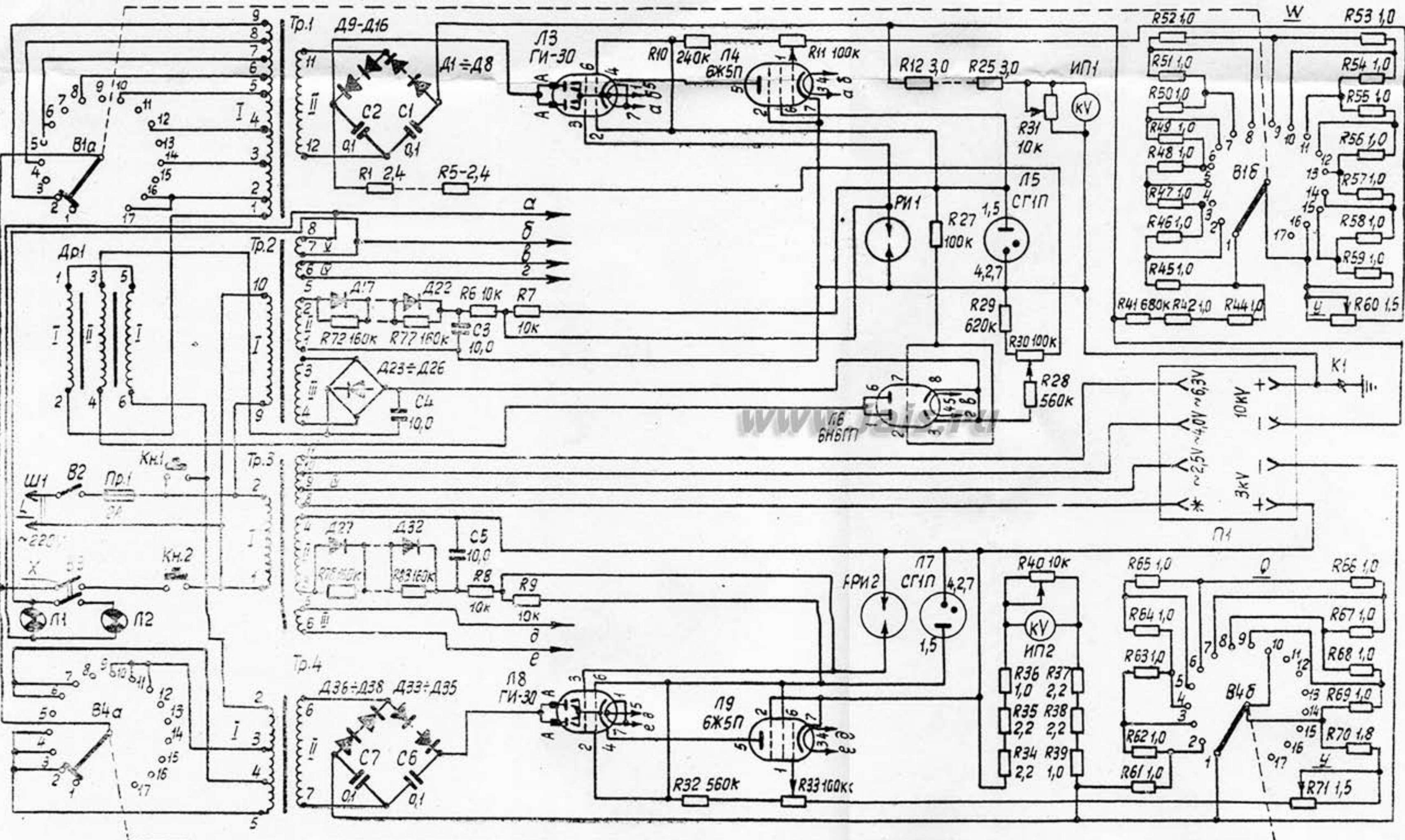
Рис. 2. Принципиальная схема ВИС-23
