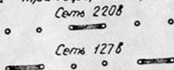
Схема переключения перемычек клеммной панели трансформатора
