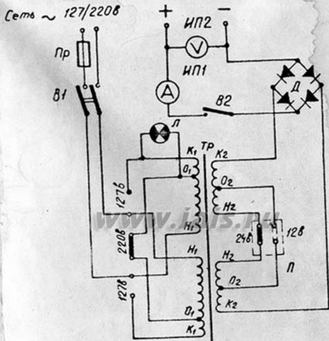
Схема переключения перемычек клеммной панели трансформатора
