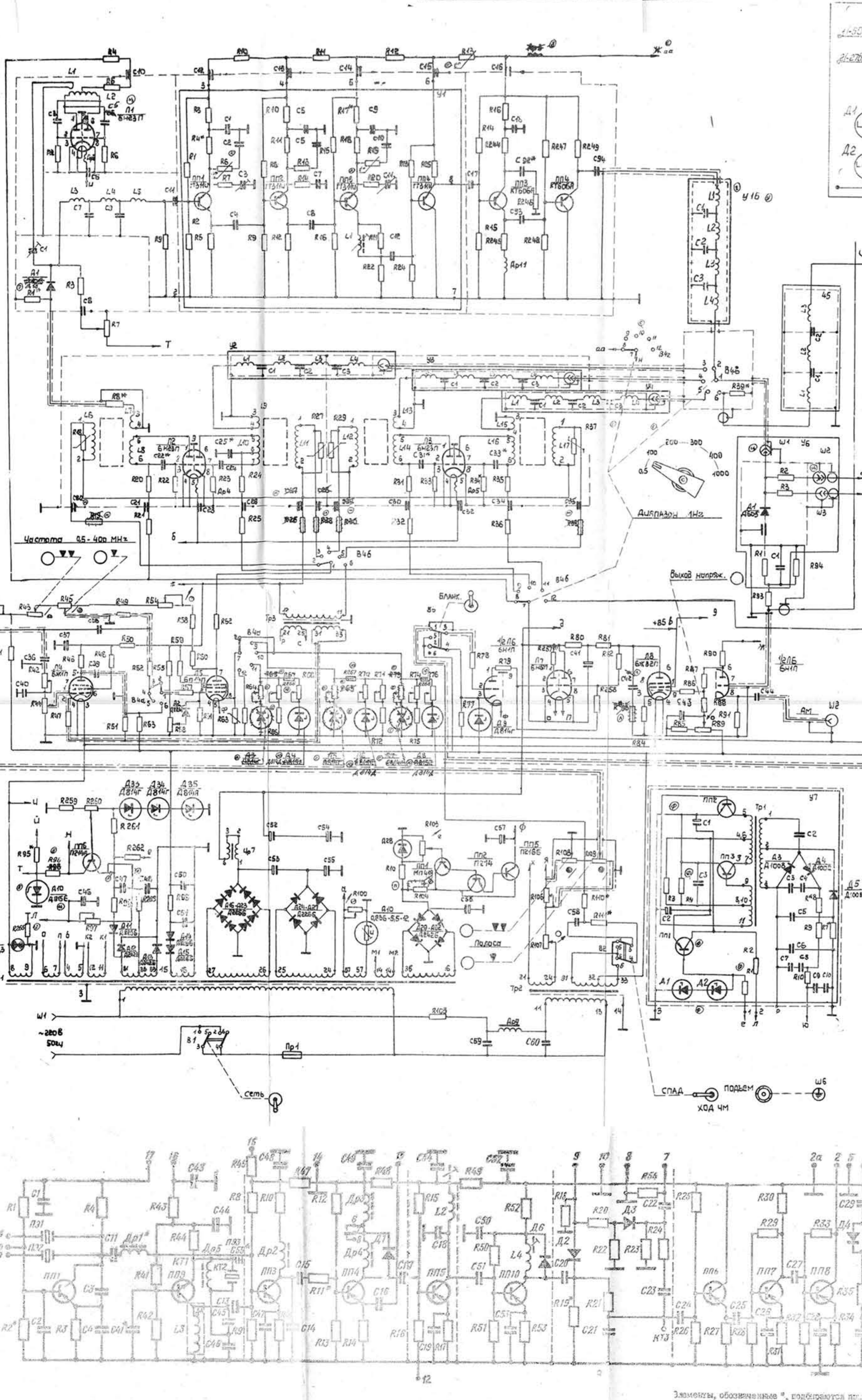
Рис. 12. БЛОК МЕТКО 2.248.009 СЗ
