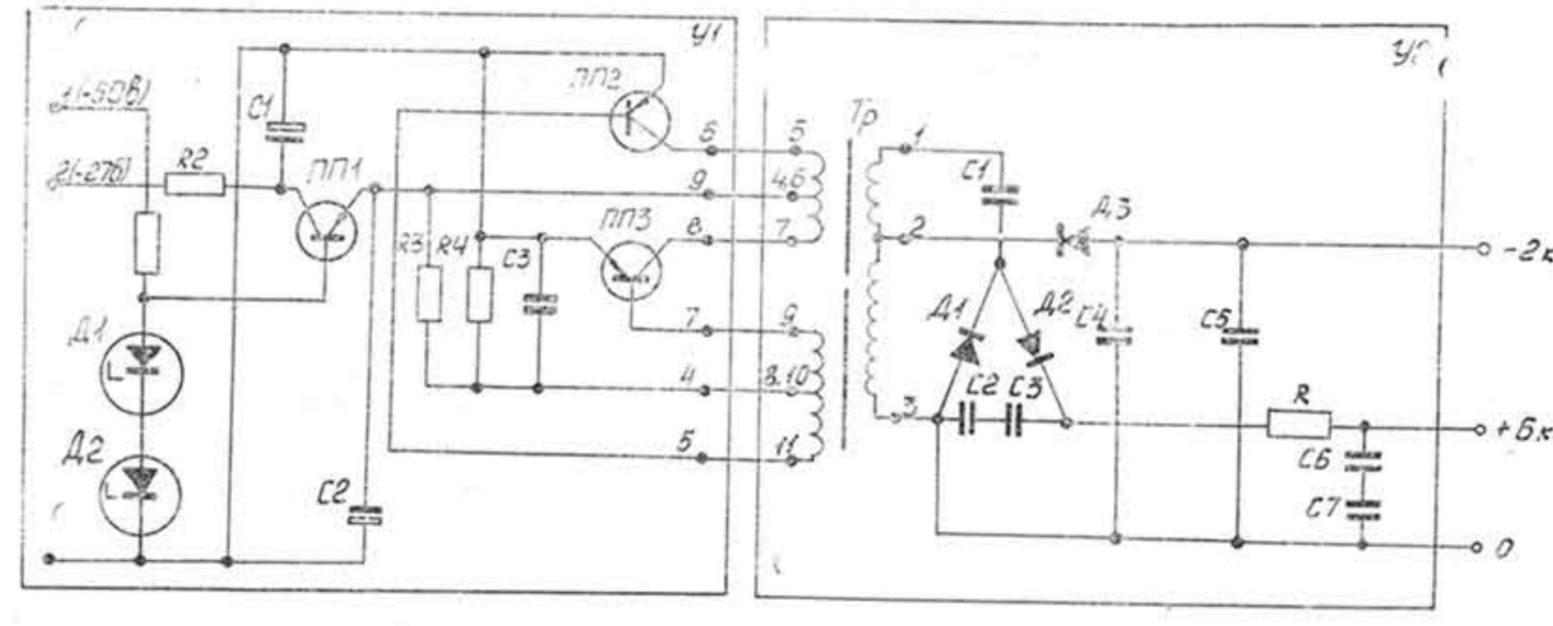
Рис. 13. Высоковольтный источник питания. 2.087.156-1 СхЭ
