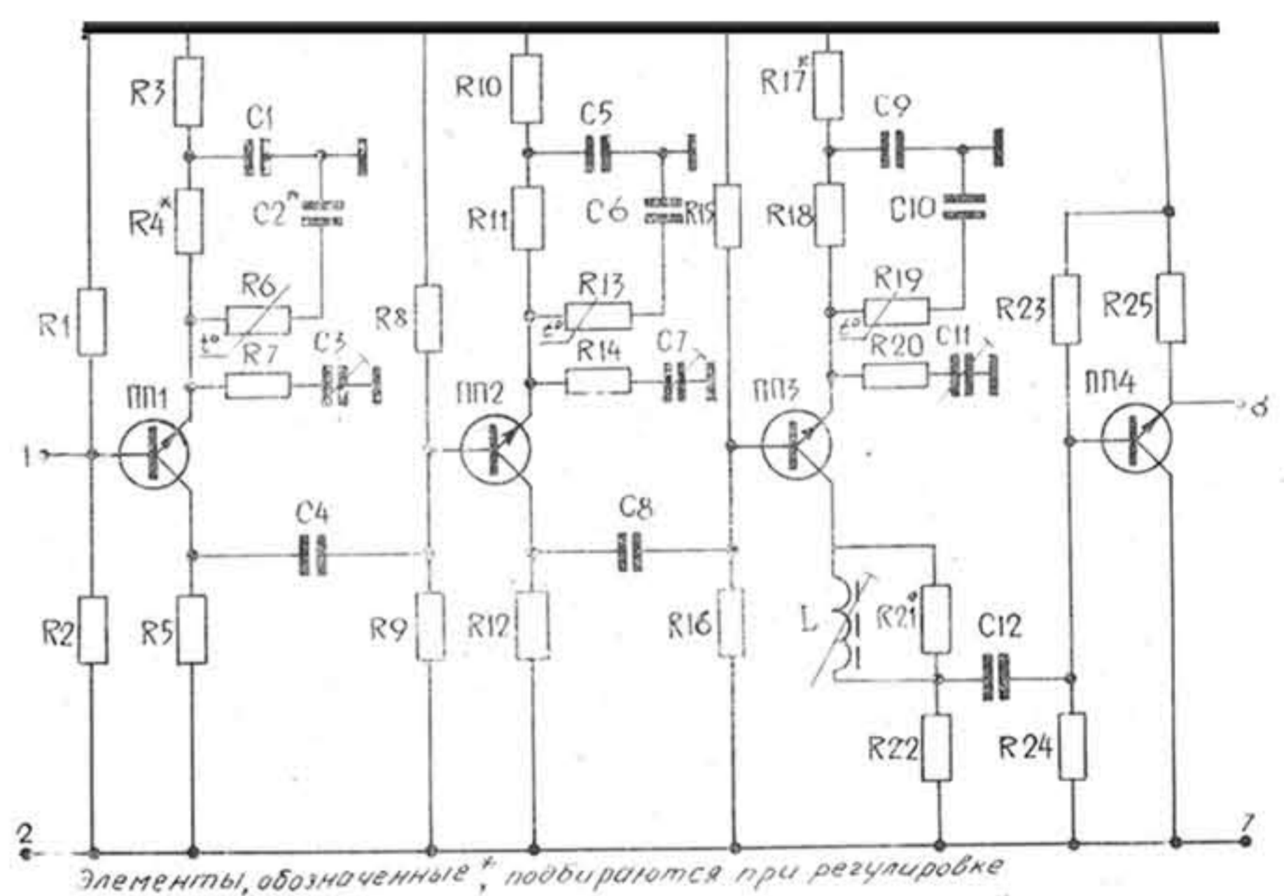
Рис. 11. Четырехкаскадный усилитель 2.030.014-1 СхЭ
