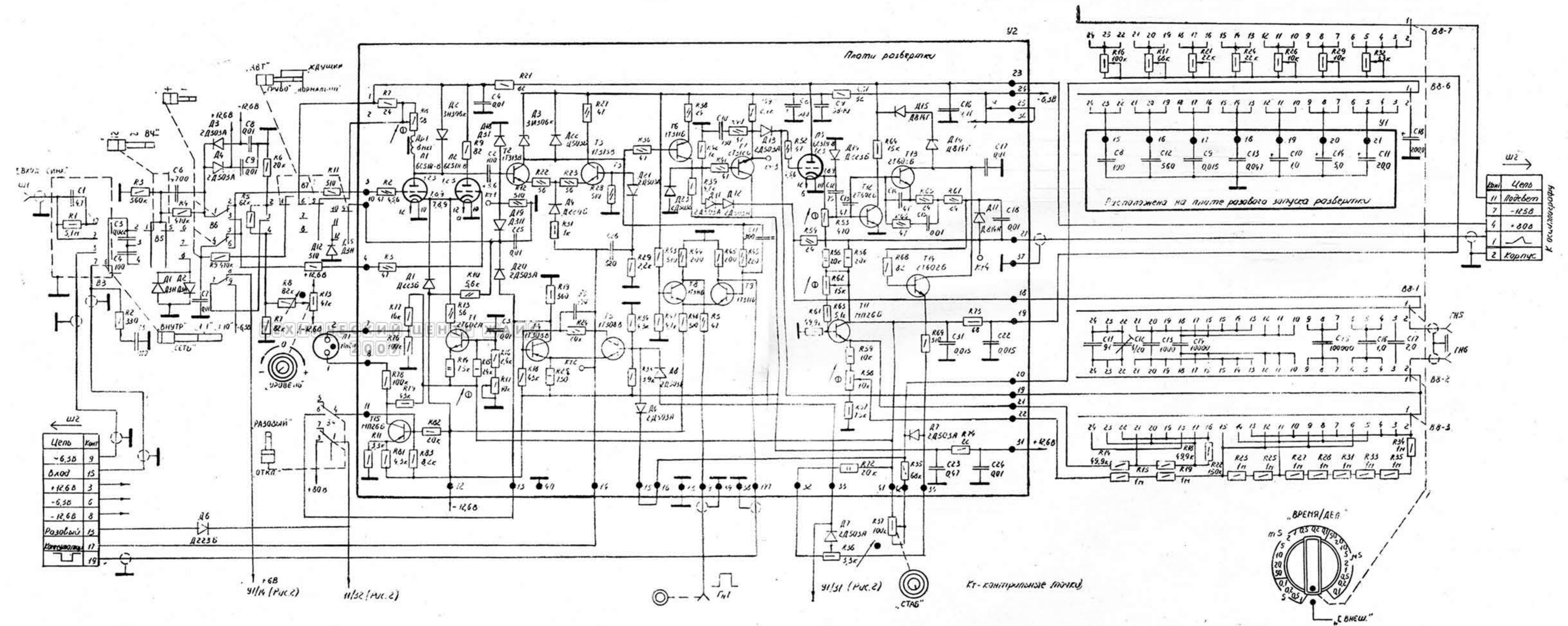
Рис. 1. Схема развертки
