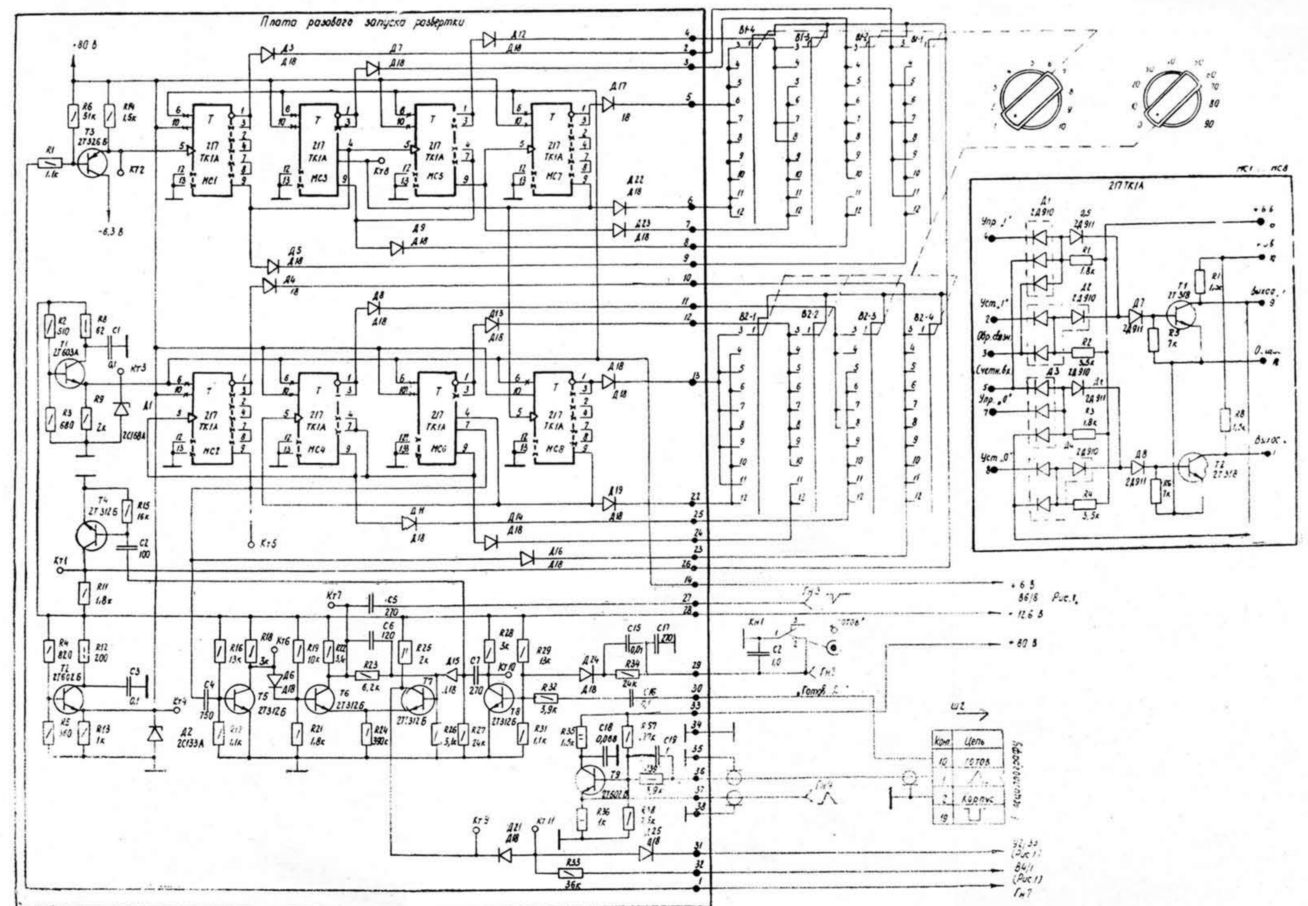
Рис. 2. Схема разового запуска развертки
