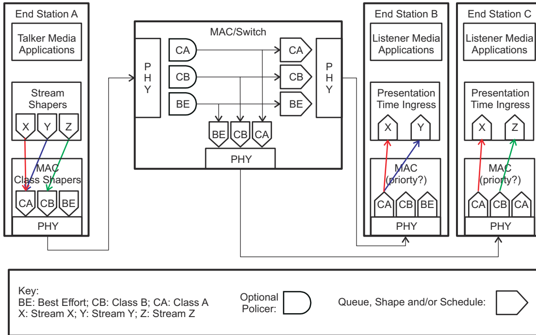
Figure 13-105. AV Stream Queuing/Policing
