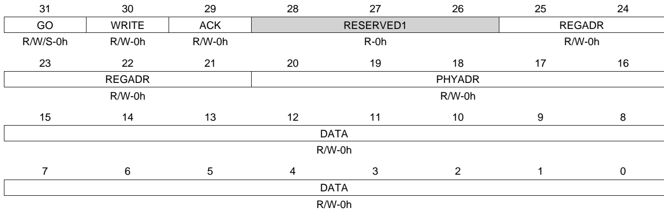
Figure 15-246. MDIO_USERACCESS1 Register
