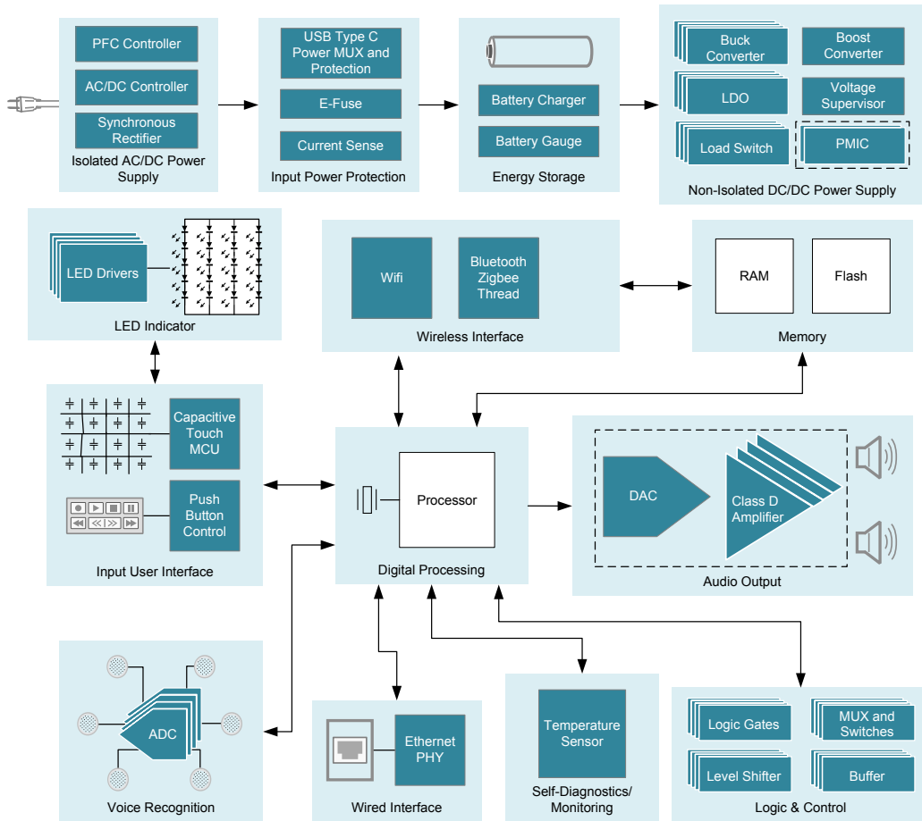
그림 2. TI의 스마트 스피커 시스템 블록 다이어그램.
