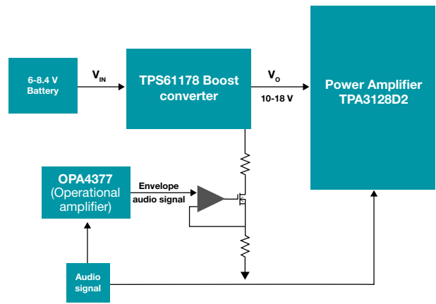
그림 5. 엔벨로프 트래킹 전원 공급 장치 레퍼런스 디자인.
