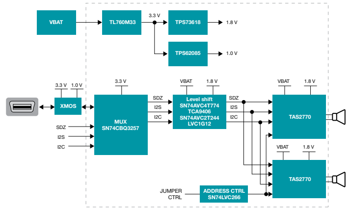
그림 4. 스테레오 평가 모듈 레퍼런스 디자인.
