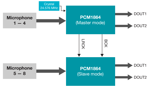
그림 3. 원형 마이크 보드 레퍼런스 설계.
