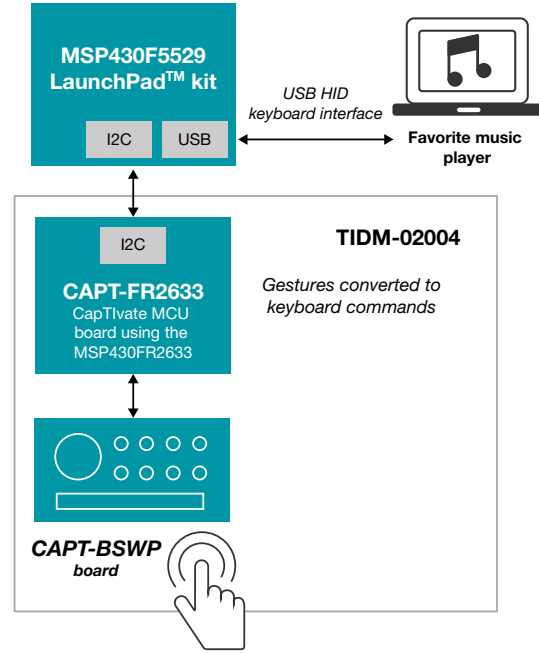
그림 7. 제스처 기반 정전식 터치 인터페이스 레퍼런스 설계.
