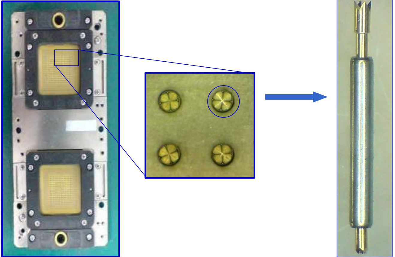
Pogo Pin
