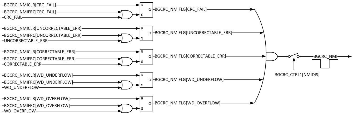
Figure 7-3. BGCR_C NMI
