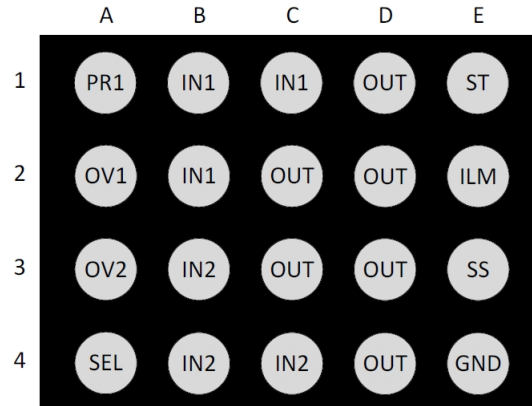
TPS2124 (YFP) Package 20-Pin WCSP Bottom View
