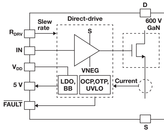
圖 16。LMG3410 整合驅動器、保護與監控功能與 GaN 開關。
