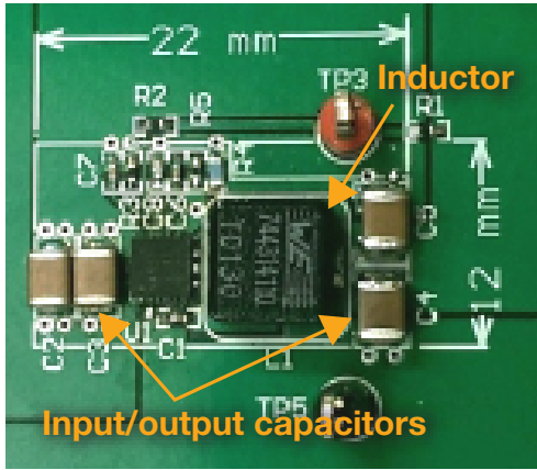
圖 4。電感器和電容器等被動元件可佔用大量空間。
