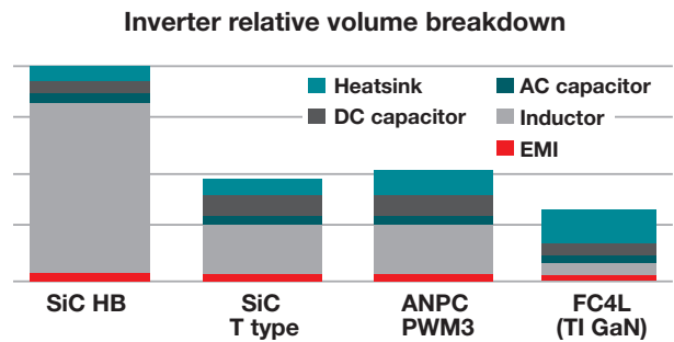
圖 15。與各種拓撲與開關類型的整體體積相比，TI 的 FC4L GaN 解決方案提供之功率密度最為優異。
