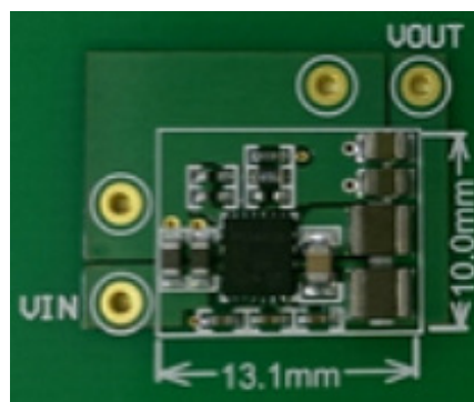
圖 3•10A 負載點轉換器測量值 面積為 13.1 mm 乘以 10 mm，進而產生 76 \text{ mA/mm}^2 電流密度。
