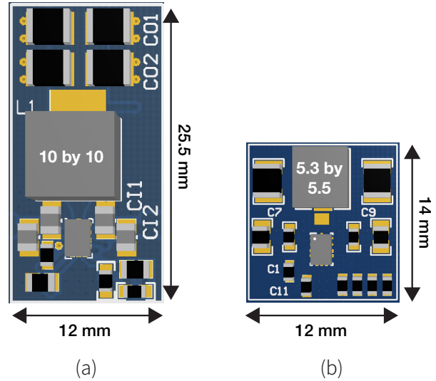
圖 5。3A、36V 轉換器在 400 kHz (a) 與 2 MHz (b) 下切換時的尺寸比較。
