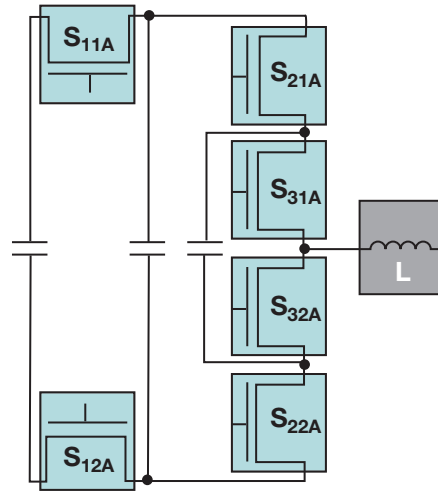
圖 14。採用 GaN 開關的飛馳電容四級轉換器拓撲。
