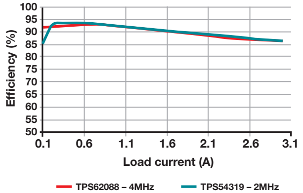
圖 7。比較 3.3V 至 1.8V 降壓轉換器的 DC/DC 效率。TPS54319 採用 TI 之前的電源處理節點，並在 2 MHz 下進行切換；TPS62088 則使用 TI 最新電源處理和經過改良的切換 FoM，並在 4 MHz 下切換。
