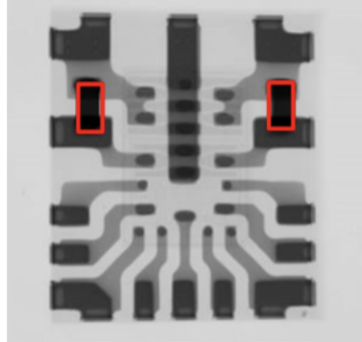
圖 17。LMQ61460-Q1 的 X 光攝影，並強調整合式旁路電容器。
