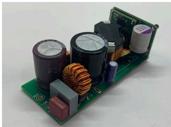
圖 2•65W 主動箝位返馳轉換器的測量值 65 mm 乘以 28 mm 乘以 25 mm。
