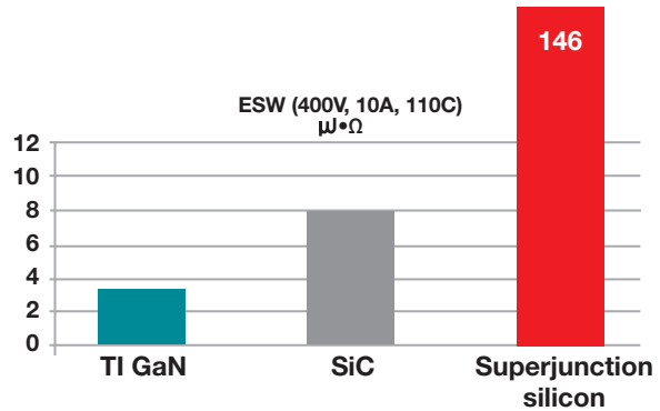
圖 8。在以 400-V 匯流排運作的情況下，GaN、SiC 與超接面矽晶切換技術的切換能量比較。TI GaN 技術可大幅降低損耗，進而提升效率。
