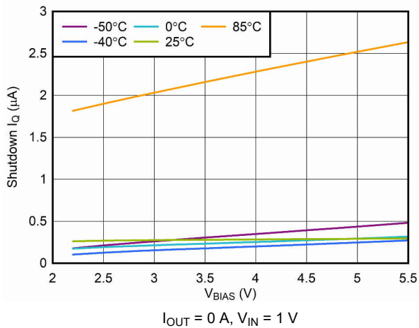
Figure 6-9. V_{\text{BIAS}} Shutdown I_Q vs V_{\text{BIAS}}
