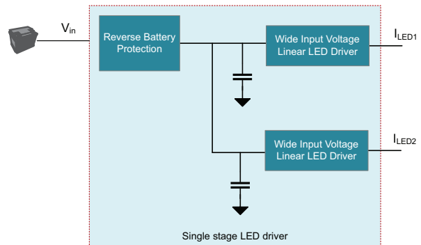
圖 8: 單級 LED 驅動器。
