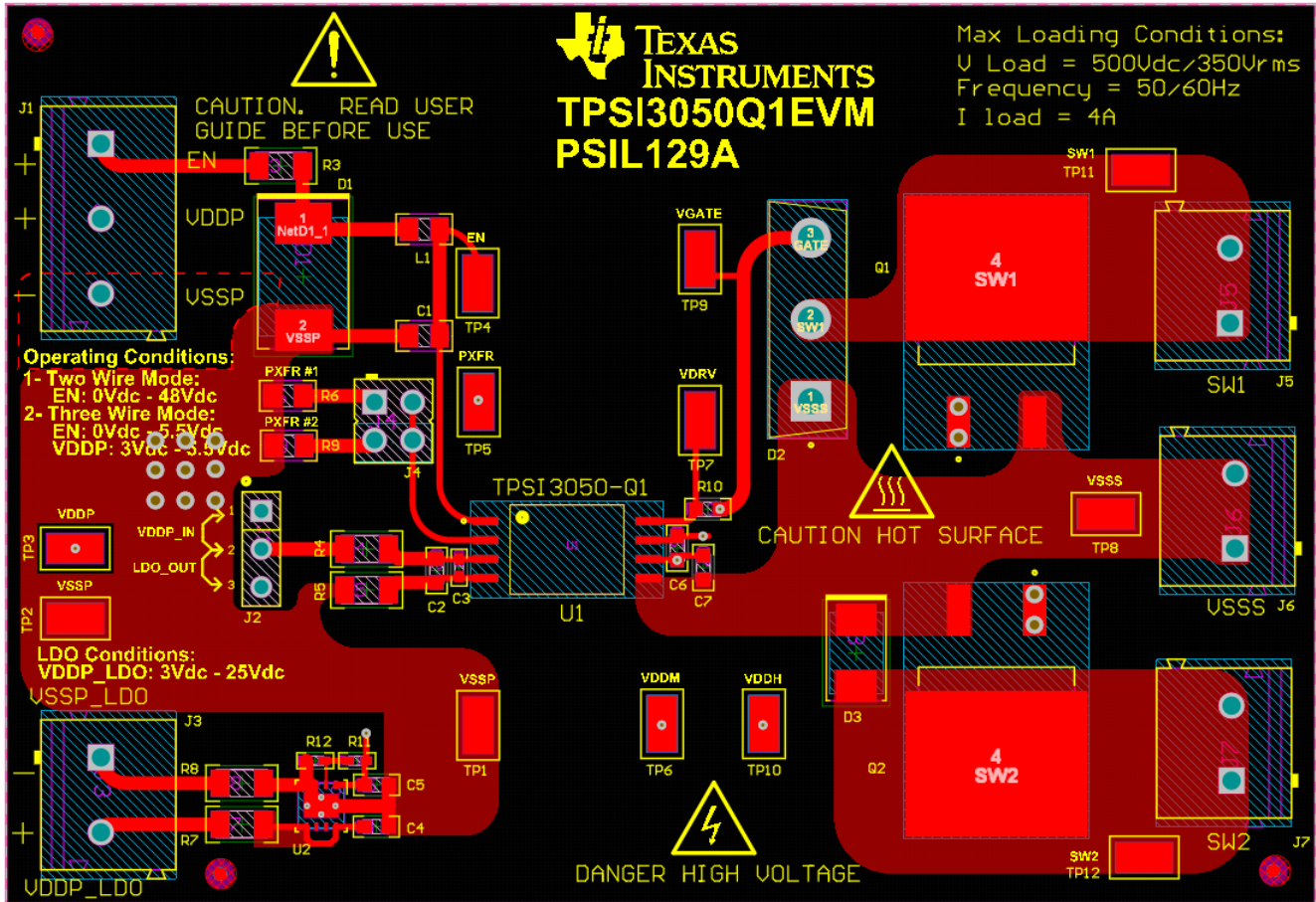
Figure 11-2. Top Layer
