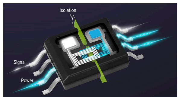
圖 8. 使用磁隔離跨隔離層可靠地傳送電源和訊號。
