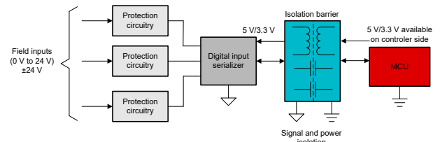
圖 13. PLC 數位輸入模組與隔離資料和功率。
