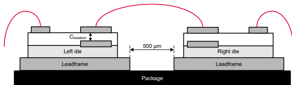
圖 6. 電容性隔離器範例。
