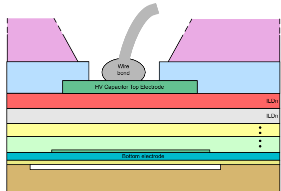
圖 7. Example cross-section of TI 的高壓隔離 SiO 2 電容器的截面積範例。
