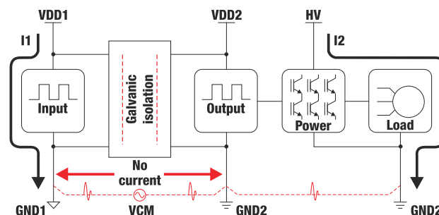
圖 1. 低至高電壓電氣訊號隔離。
