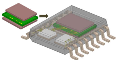
圖 9. 磁耦合鍍鐵氧體高性能變壓器。
