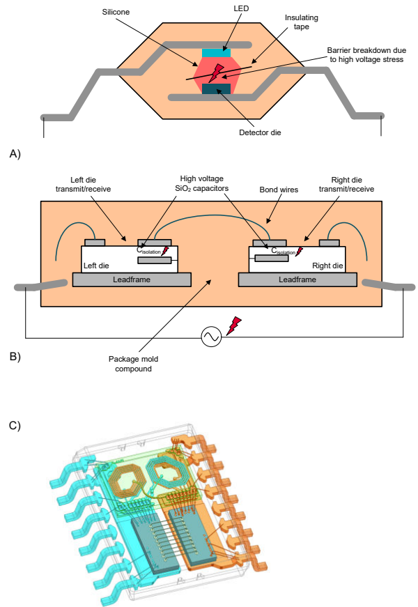
圖 4. 半導體隔離技術：光耦合器 (a)；電容式 (b)；變壓器 (c)。
