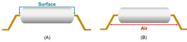
圖 3. 跨表面的爬電距離和通過隔離器封裝的空氣間隙。
