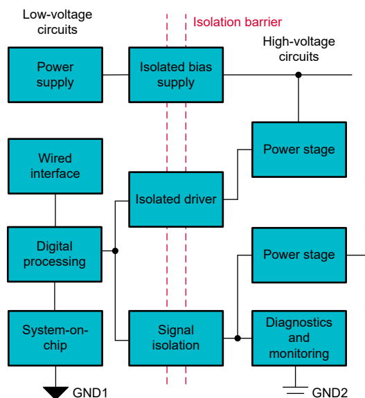
圖 2. 通過隔離層傳輸的訊號類型。
