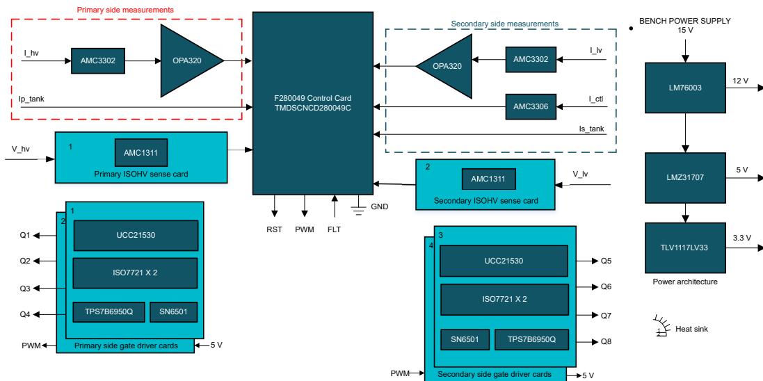
圖 12. 雙向雙有源電橋參考設計配置圖。
